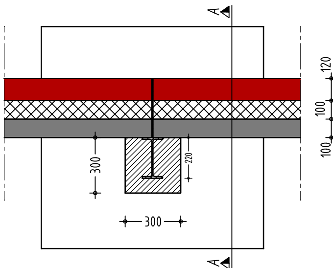
Bovenaanzicht langswand
