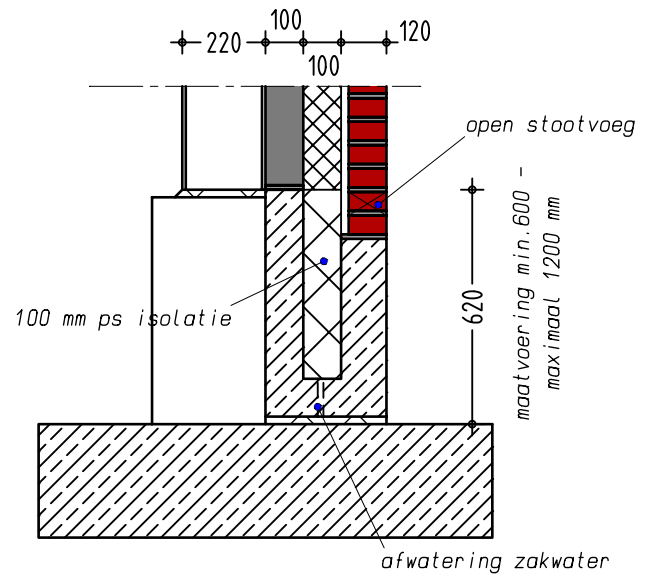
Doorsnede AA
