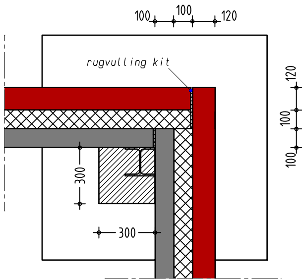
Bovenaanzicht hoek
